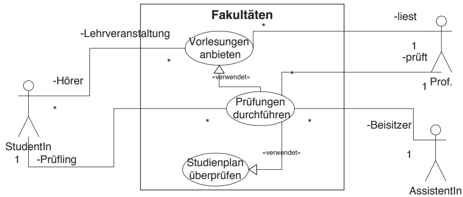
Abbildung 1.27: Identifizierung von Anwendungsfällen und Akteuren
