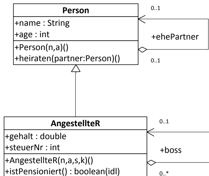
Abbildung 3.2: Die Generalisierung/Spezialisierung
