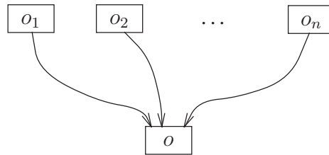
Abbildung 1.15: Gemeinsames Unterobjekt
