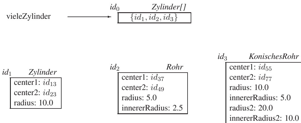
Abbildung 3.12: Objektbank mit einem Zylinder[] -Objekt
