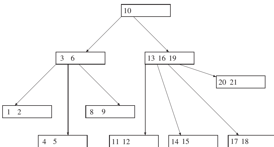
Abbildung 7.15: Löschen der 7
