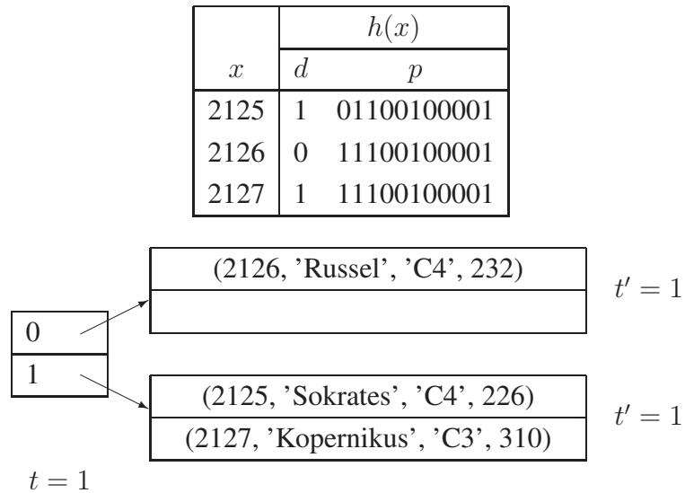
Abbildung 8.8: Ein Hash-Index
